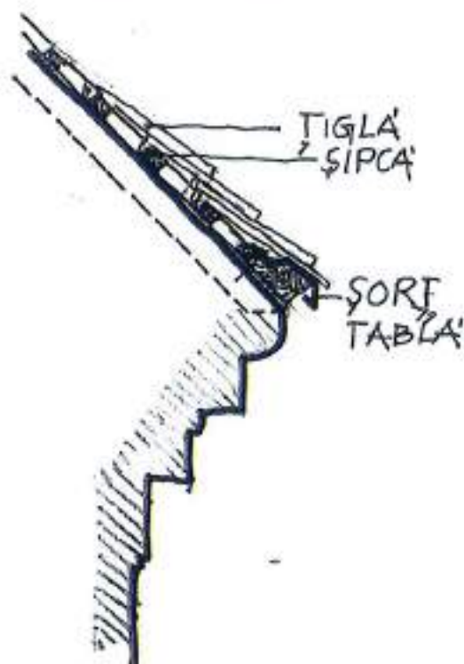
Fig. 7.- Schiță cu rezolvarea cornișei turnului prin montarea unei scânduri cu un șorț de tablă inoxidabilă.
