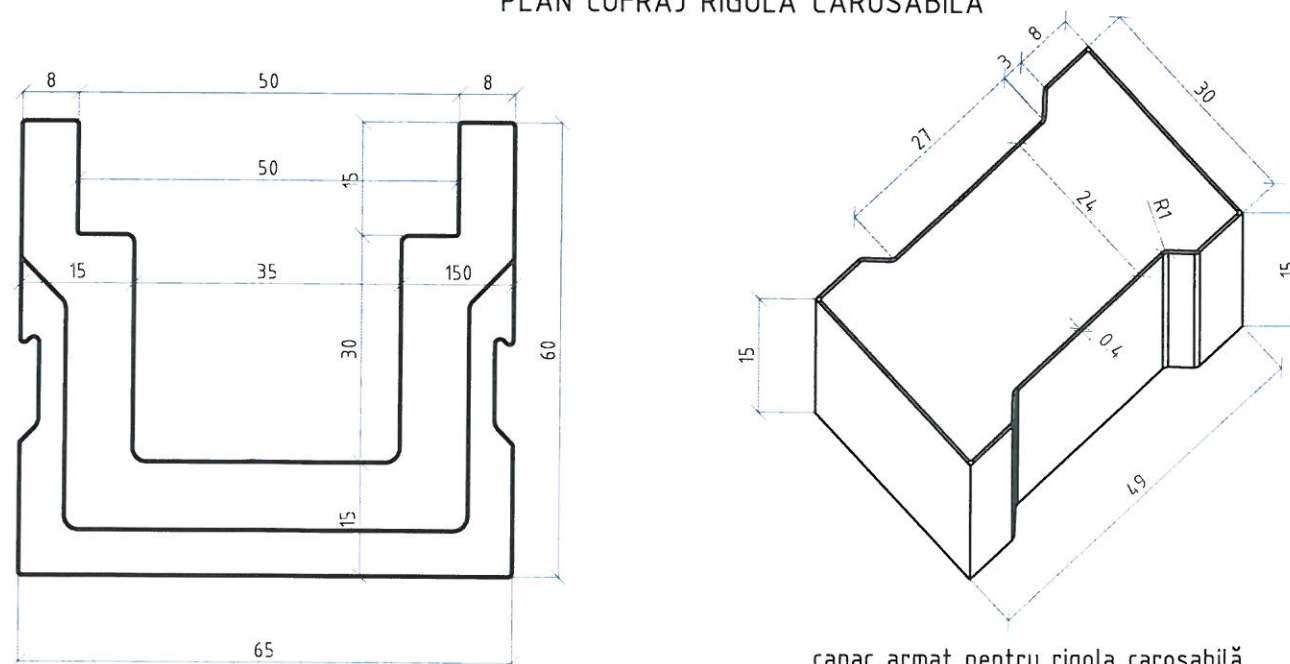
PLAN COFRAJ RIGOLĂ CAROSABILĂ
