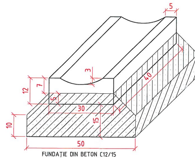
Detaliu rigolă tip scafă scara 1:10
