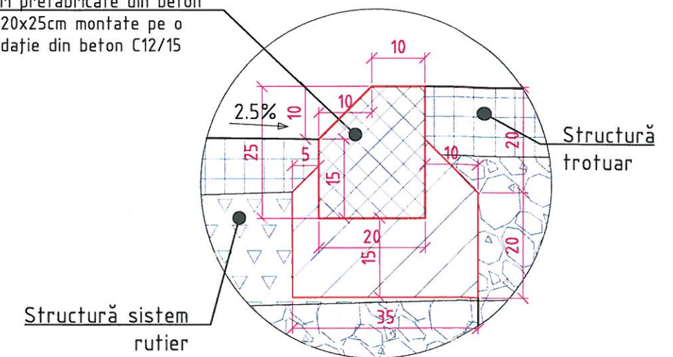
Detaliu bordură 50x20x25 scara 1:10
