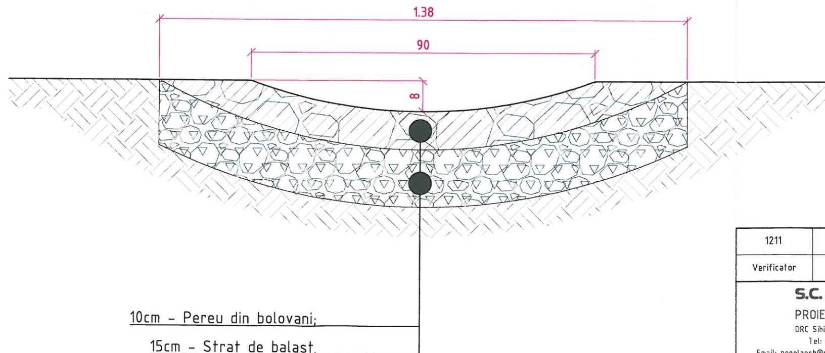
Detaliu șanț pereat scara 1:10
