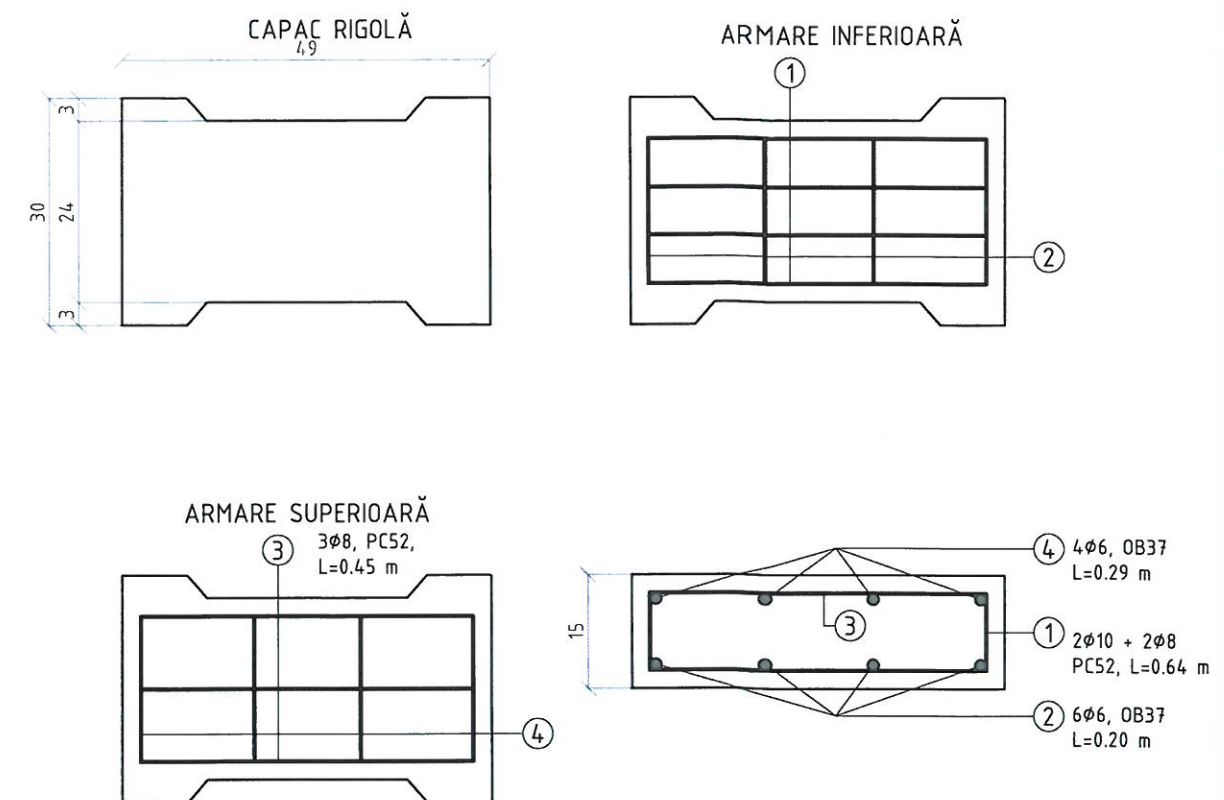
PLAN ARMARE RIGOLĂ CAROSABILĂ
